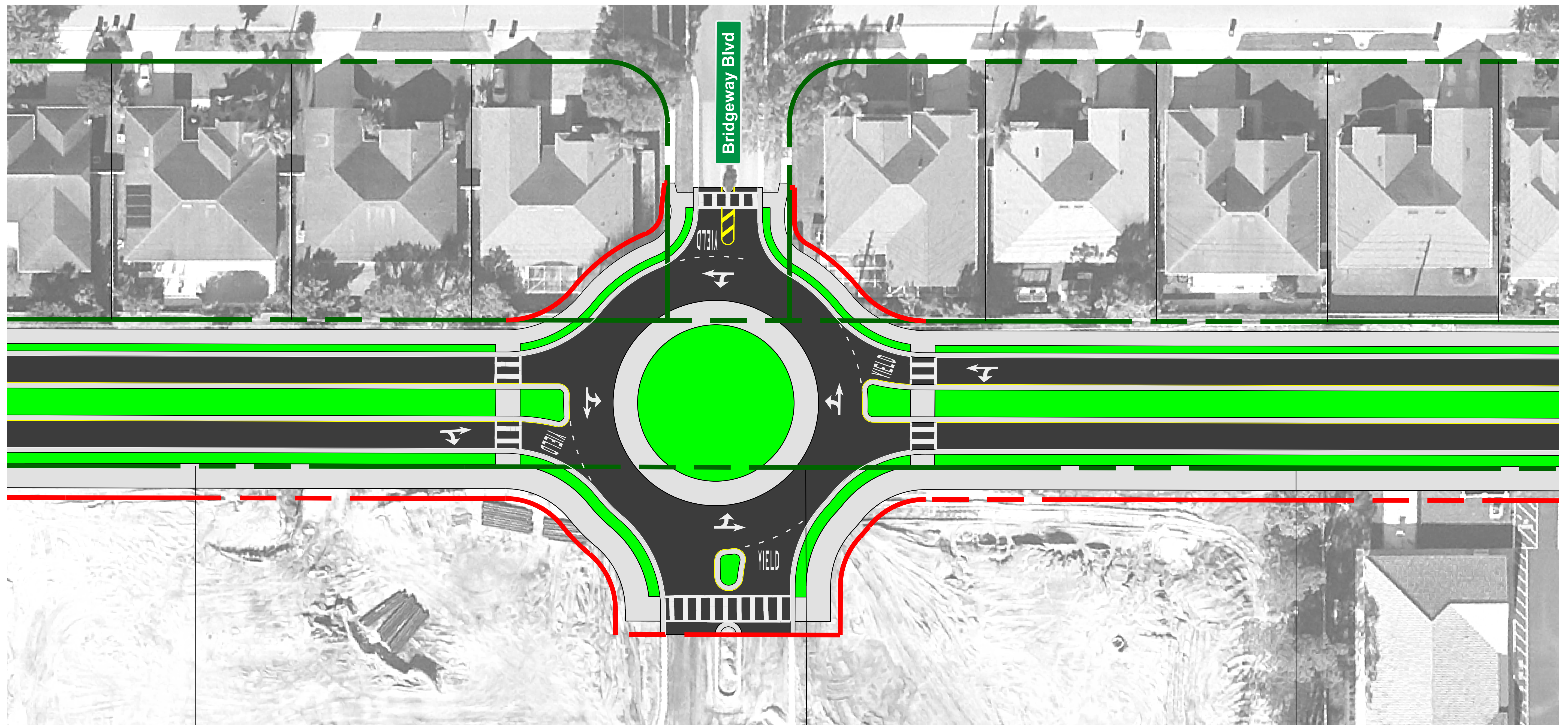
Mini Roundabout at Bridgeway Blvd.
